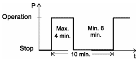
图7. 间歇运行
